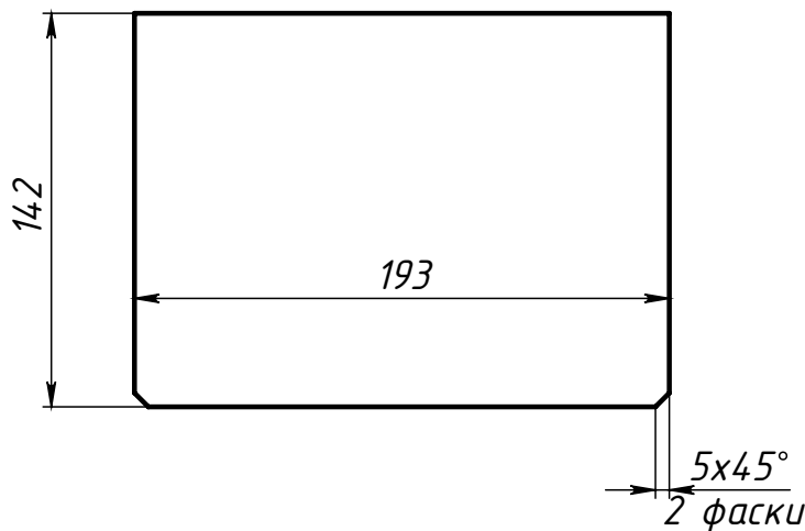
Поз.2 (Ребро)
